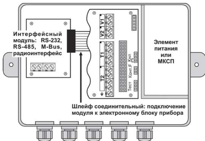
Рисунок Б.3 – Внешний вид монтажного отсека вычислителя КА-РАТ-306 с установленным интерфейсным модулем
