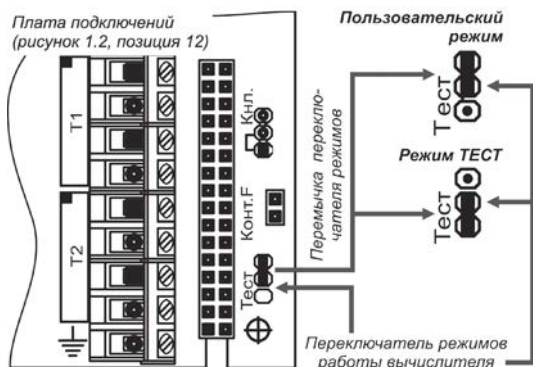
Рисунок 2.4 – Установка режимов работы вычислителя
